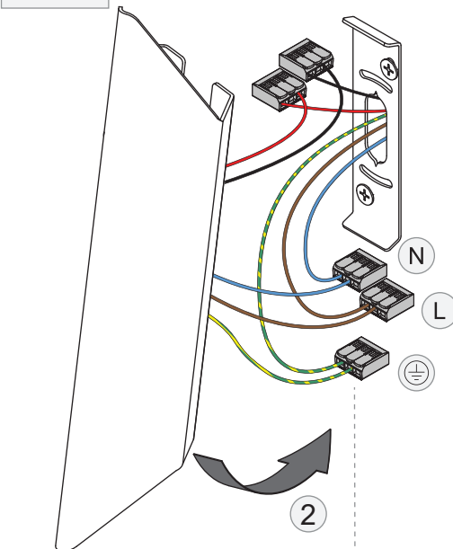
2.a DALI DIAGRAM
