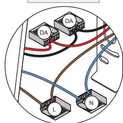
2.a DALI DIAGRAM
